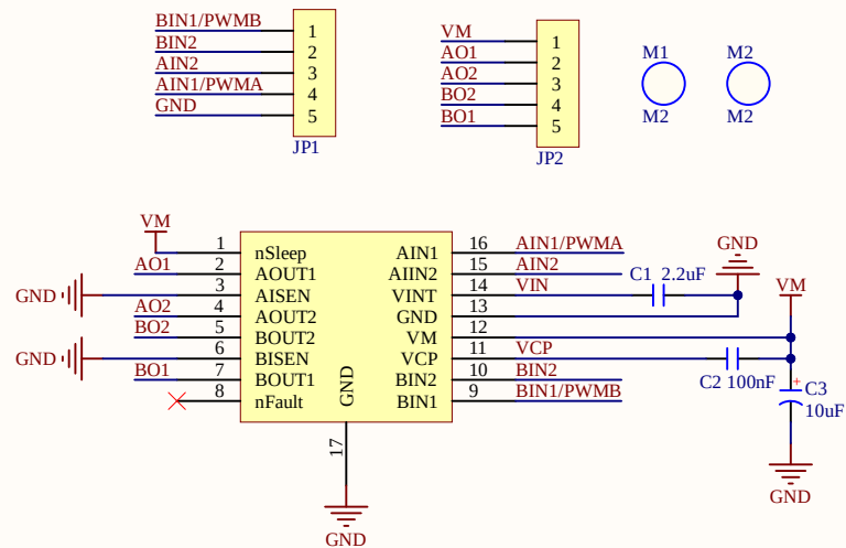
电机驱动模块
