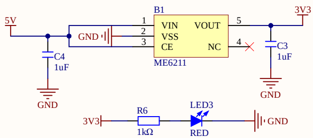
3V3线性稳压
