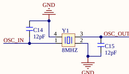
晶振电路
