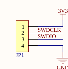
下载电路
