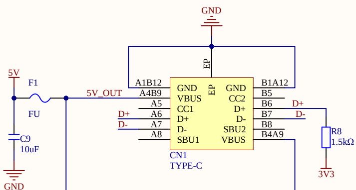
TYPE-C接口电路
