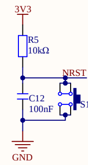
复位电路
