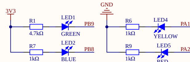
控制电路
