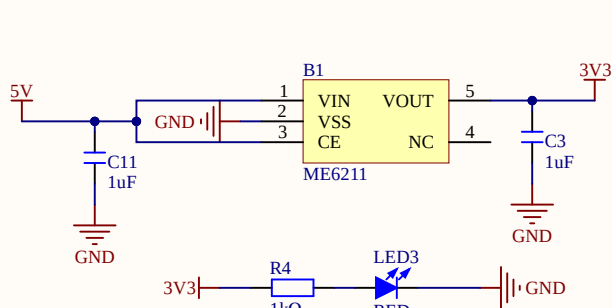
3V3稳压电路
