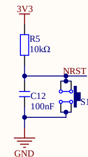
复位电路
